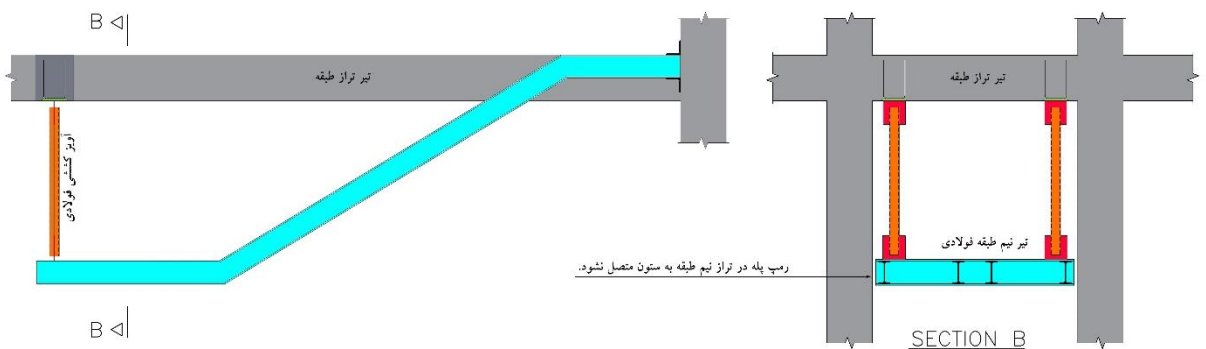
جزئیات پیشنهادی برای اتصال رمپ پله فولادی با آویز فولادی
