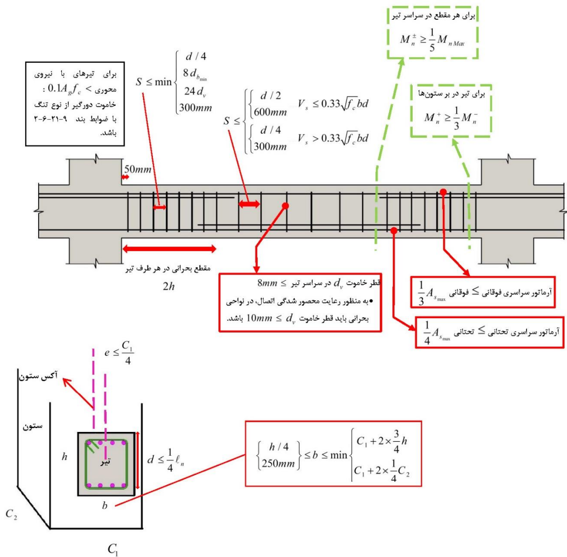
تیرهای با شکل‌پذیری متوسط
