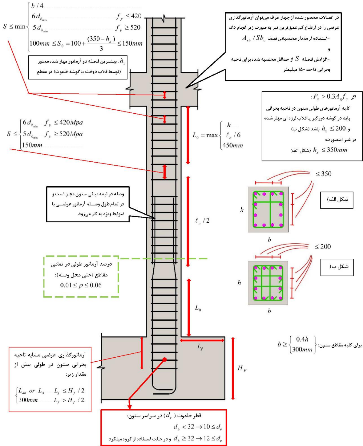
ستونهای با شکل پذیری زیاد
