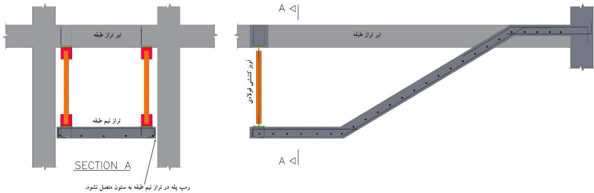
جزئیات پیشنهادی برای اتصال رمپ پله بتنی با آویز فولادی
